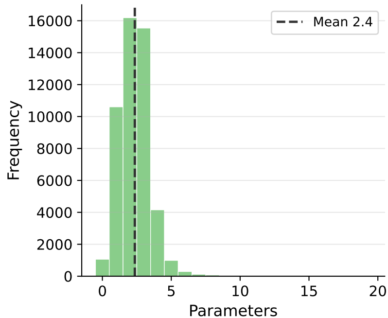
Parameters per Tool
